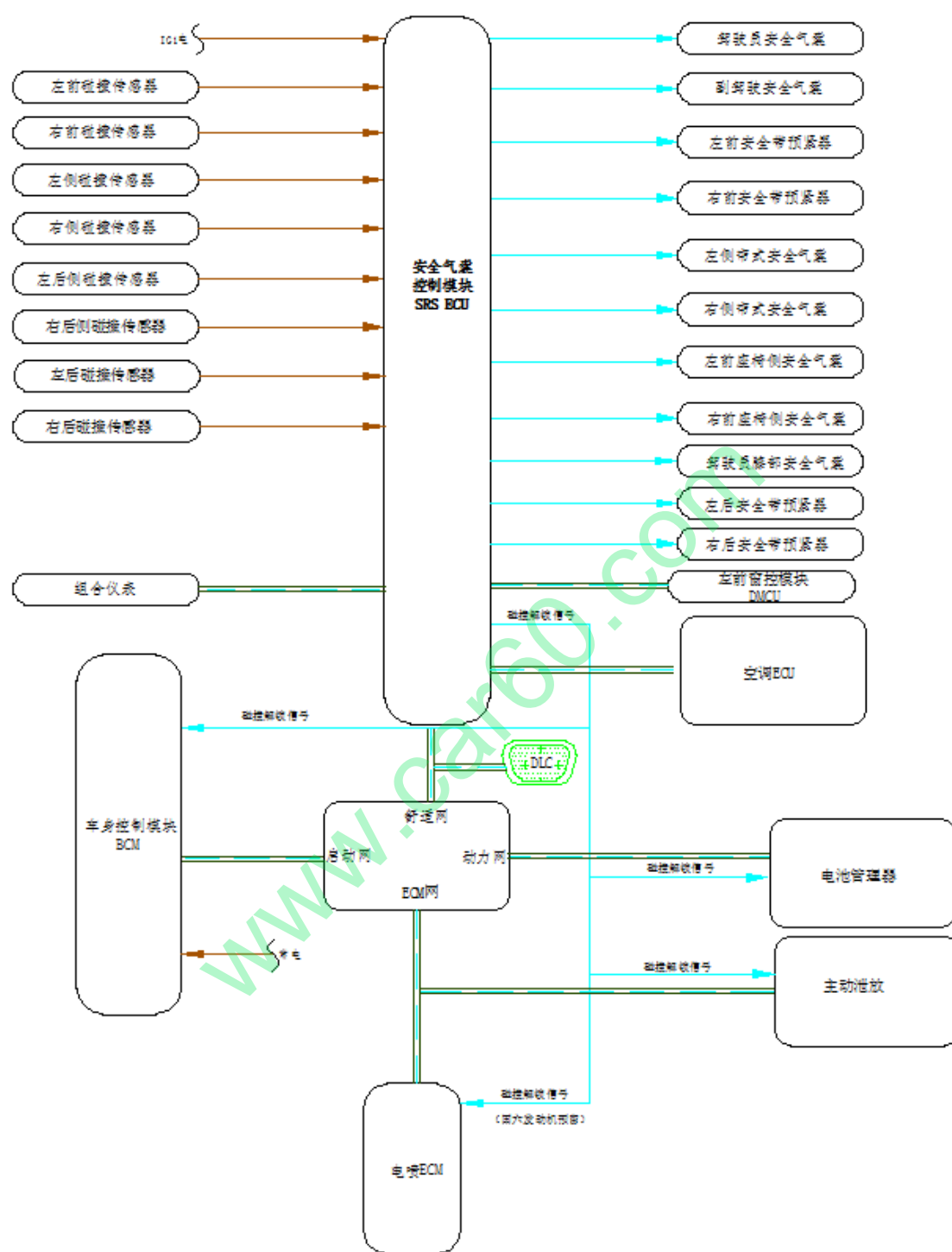
系统框图
